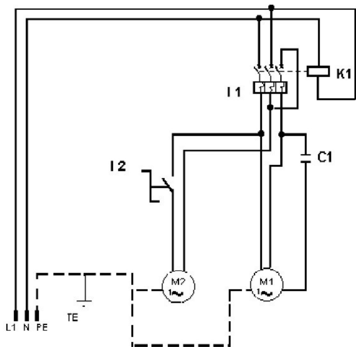
Fig. 19 - Wiring Diagram
